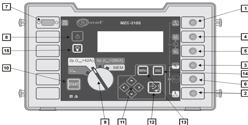
Расположение гнёзд и клавиш MZC-310S (передняя панель)
